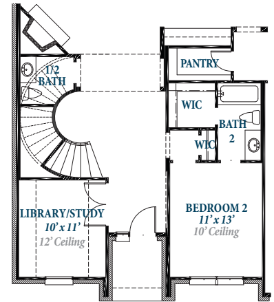
OPTIONAL HALF BATH
