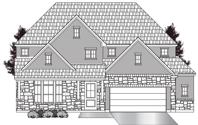
• ELEVATION D3 •
